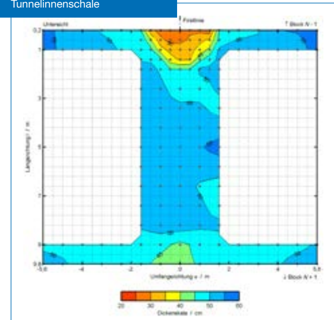
Isolinien-Darstellung der Bauteildicke eines Blocks einer Tunnelinnenschale
